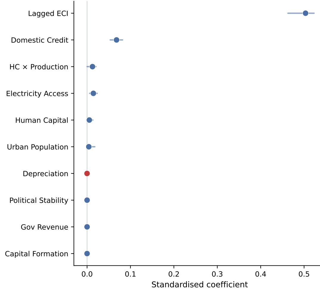
LASSO
